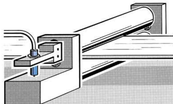
In dieser Anwendung misst der My-Com minimalste Auslenkungen der oberen Metallwalze in einer Doppelbogenkontrolle
