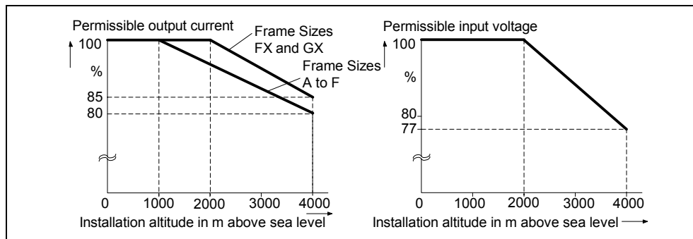
Fig. 2-3 Installation altitude
